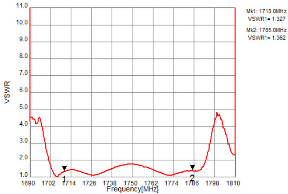
VSWR S11
